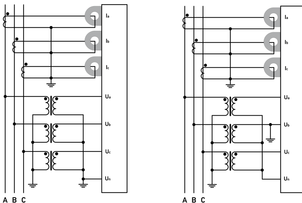
Рисунок А2.2. Схема подключения преобразователей ЭНИП-2-4X/100-24-А2Е0-32 для трехфазной трехпроводной сети: 4LN3 или 4LL3 (ЭНИП-2 настроен на измерение в режиме схемы «4-проводная»).
