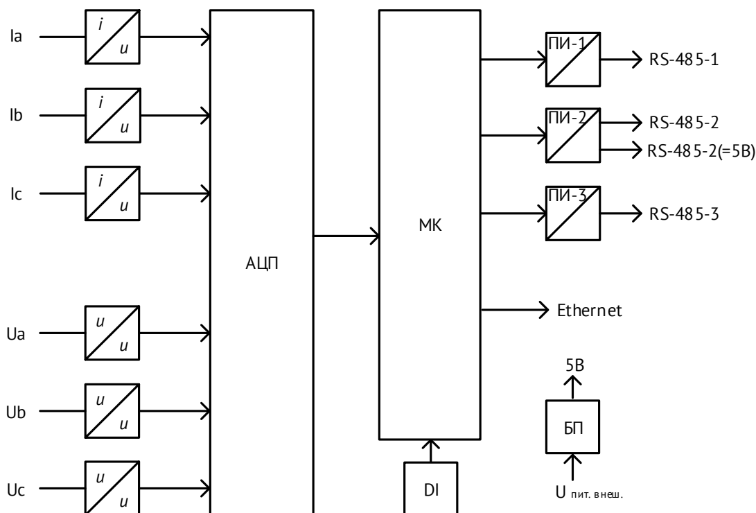
Рисунок 3.1. Структурная схема преобразователя ЭНИП-2-...-А3Е4-21
