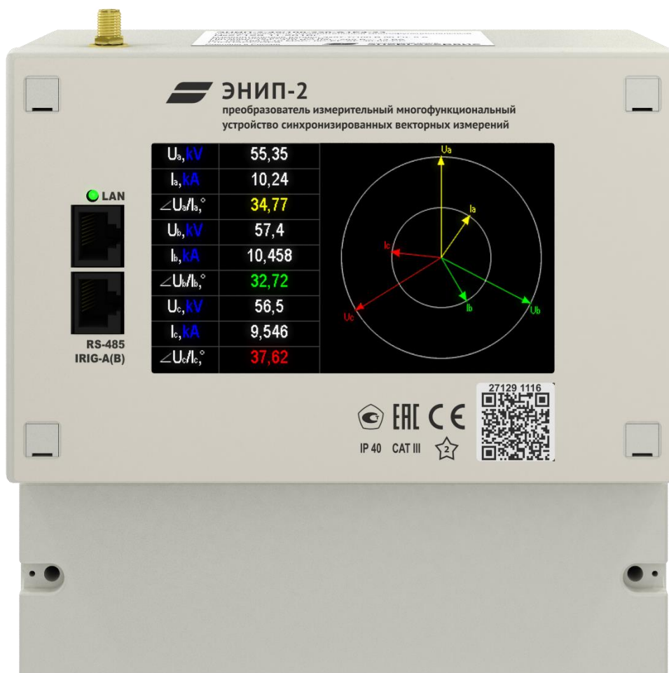
Рисунок 1.7. Модификация ЭНИП-2-...-A1E4-32
