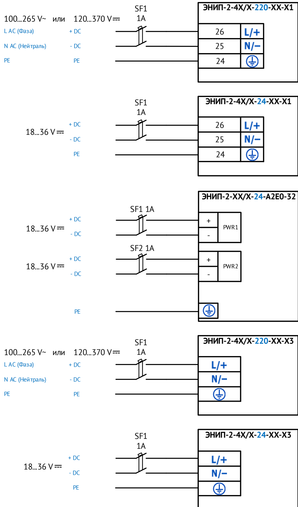
Рисунок 8.1. Схемы подключения ЭНИП-2 к цепям источника (сети) электропитания.
