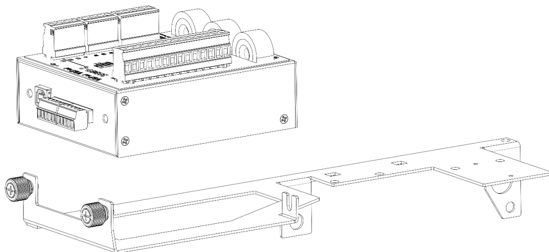
Рисунок 1.11. Способ установки преобразователя ЭНИП-2-...-32 на кронштейн RM6-KP
