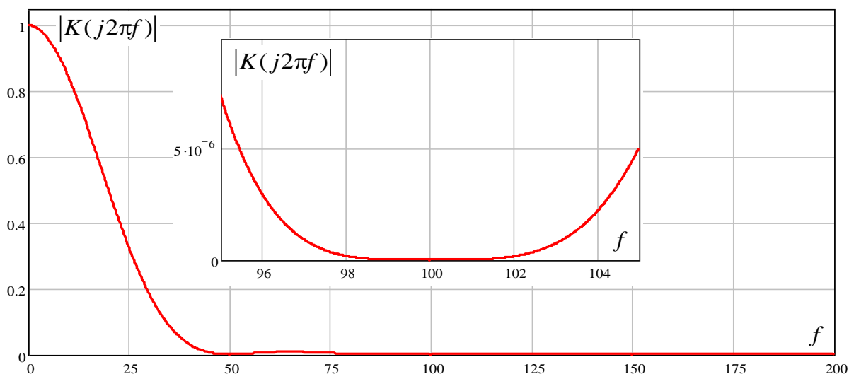
Передаточная функция аналогового фильтра-прототипа (1)
