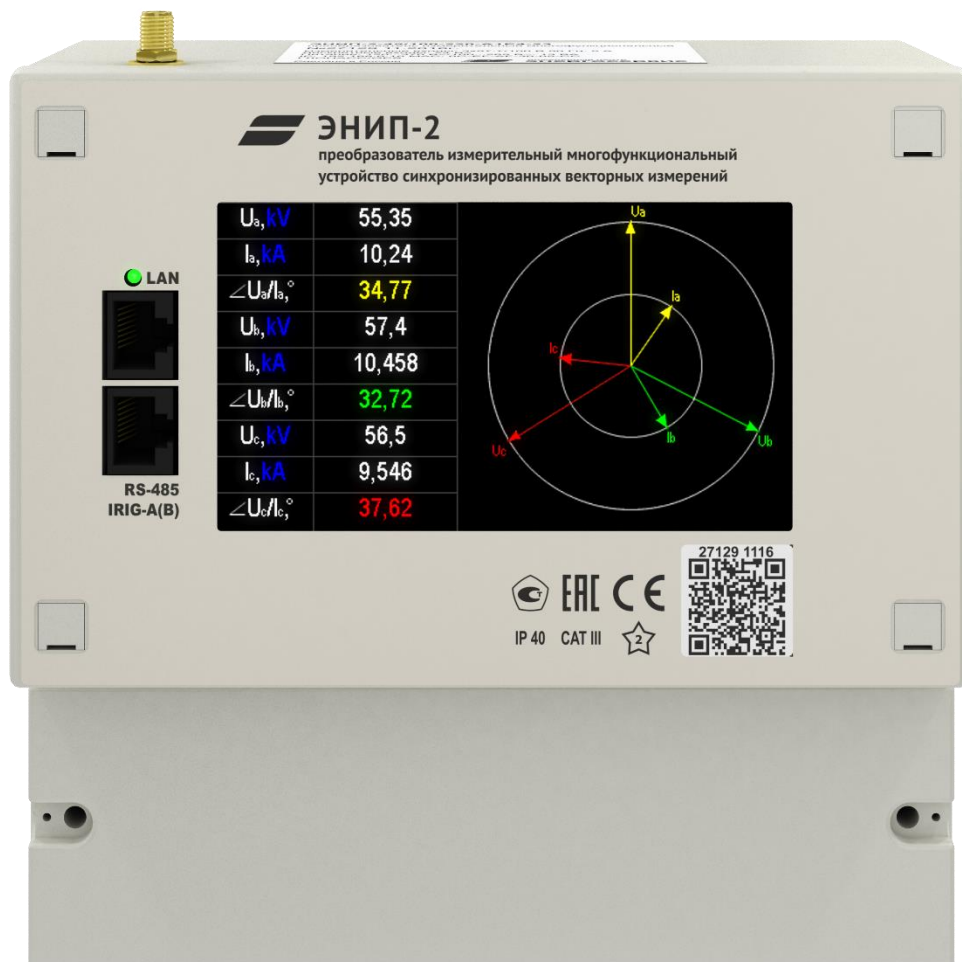
Рисунок 1.8. Модификация ЭНИП-2-0-...-A1E4-23
