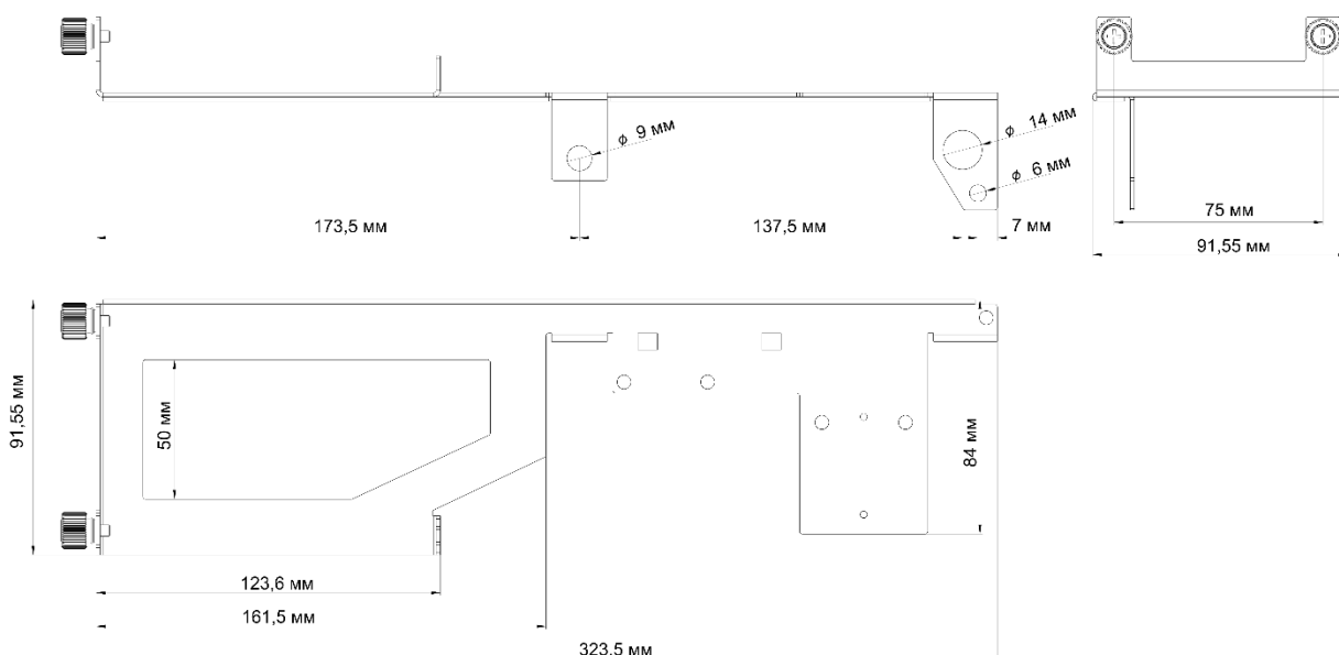
Рисунок 1.12. Габаритные размеры кронштейна RM6-KP
