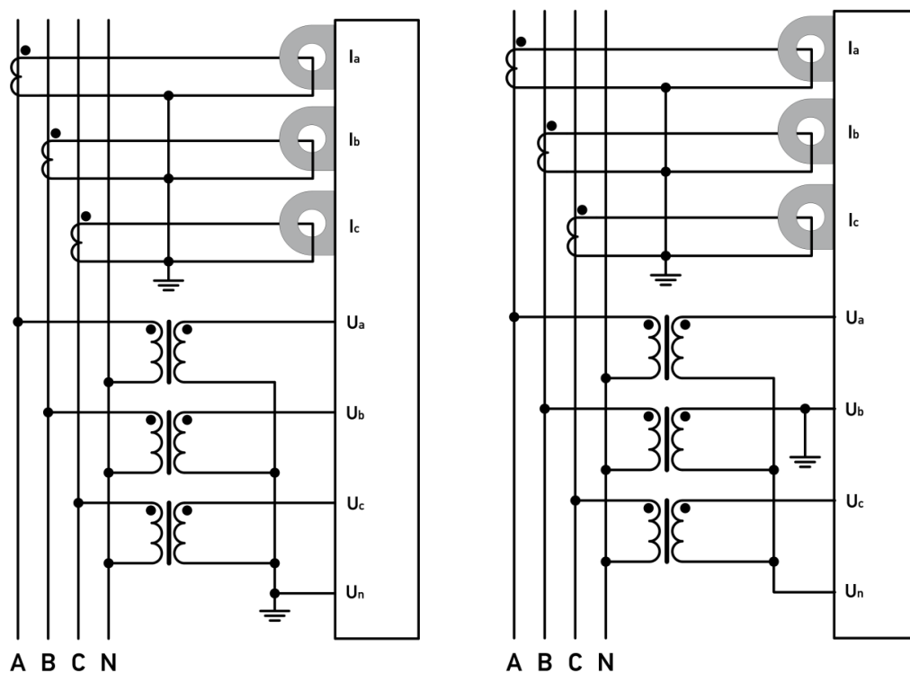
Рисунок А2.1. Схема подключения преобразователей ЭНИП-2-4X/100-24-А2Е0-32 для трехфазной четырехпроводной сети: 4LN3 или 4LL3 (ЭНИП-2 настроен на измерение в режиме схемы «4-проводная»).
