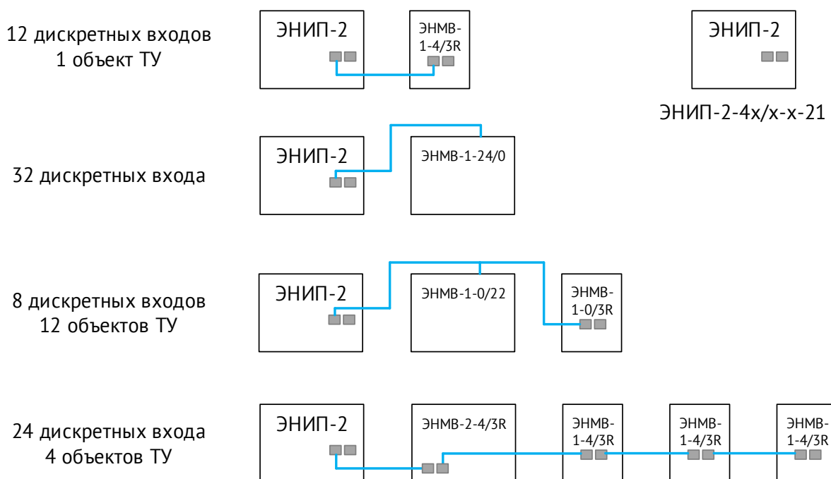
Рисунок 8.8. Примеры схем подключения ЭНИП-2-...-Х1 к внешним модулям.
