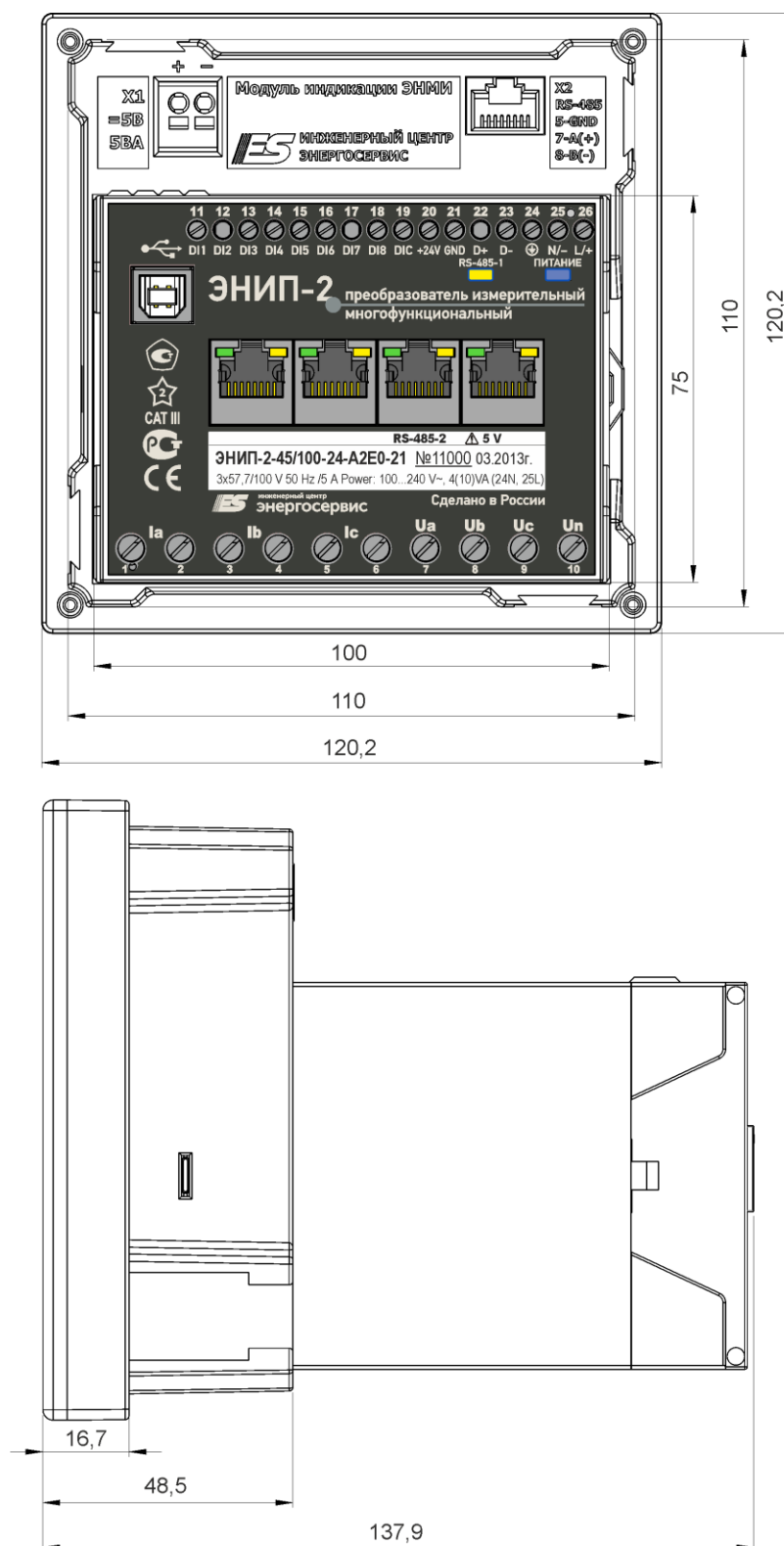
Рисунок 8.16. Габаритные размеры и схема совмещенной установки ЭНИП-2 с модулем индикации ЭНМИ, как щитового прибора.
