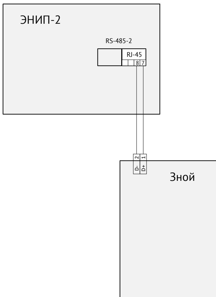
Рисунок 8.12. Подключение устройства Зной.
