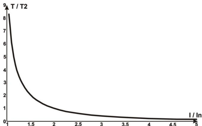
Рисунок 6 – Токо-временная характеристика
