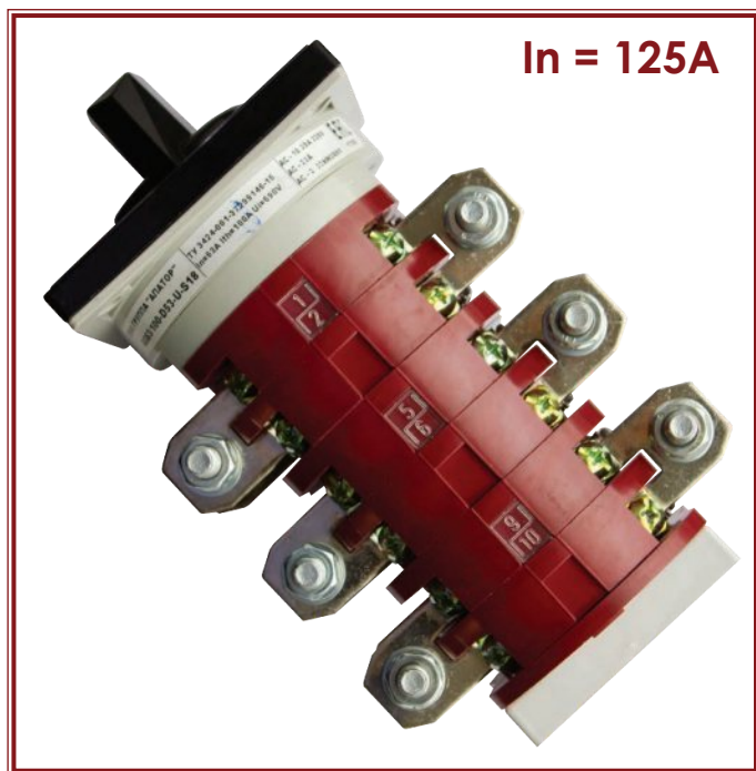
Габаритные и присоединительные размеры соответствуют группе А2.
